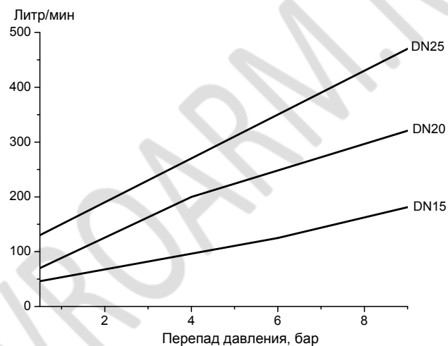
Диаграмма 1. Зависимость расхода от давления
