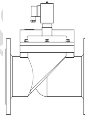
Рисунок 1. Устройство
